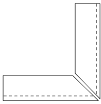
ÁNGULO PELDAÑO 120. EXT. ANTISLIP 120 x 32 x 45/3 (G 46 x 2) 48" x 12,5" x 17,7"/1"
