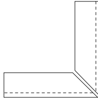
ÁNGULO PELDAÑO 120. EXT. 120 x 32 x 45/3 (G 46 x 2) 48" x 12,5" x 17,7"/1" ♦
